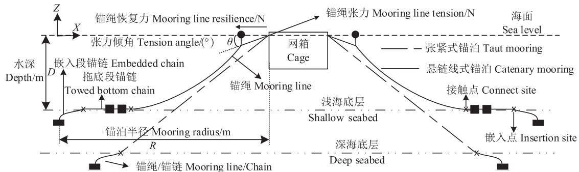
图2 张紧式与悬链线式锚泊系统
