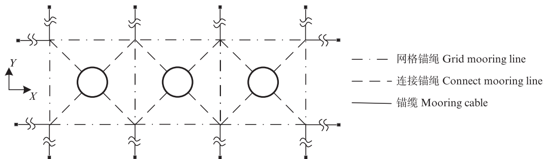
图4 养殖网箱阵列锚系分布
