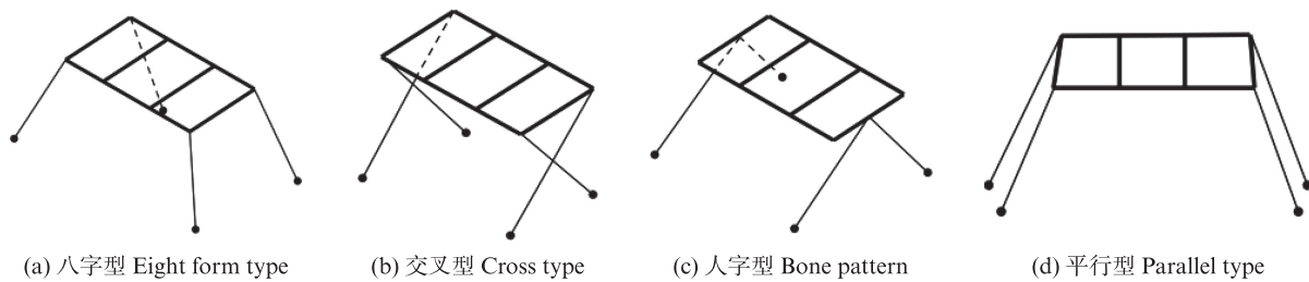
图3 多点锚泊不同布链方式
