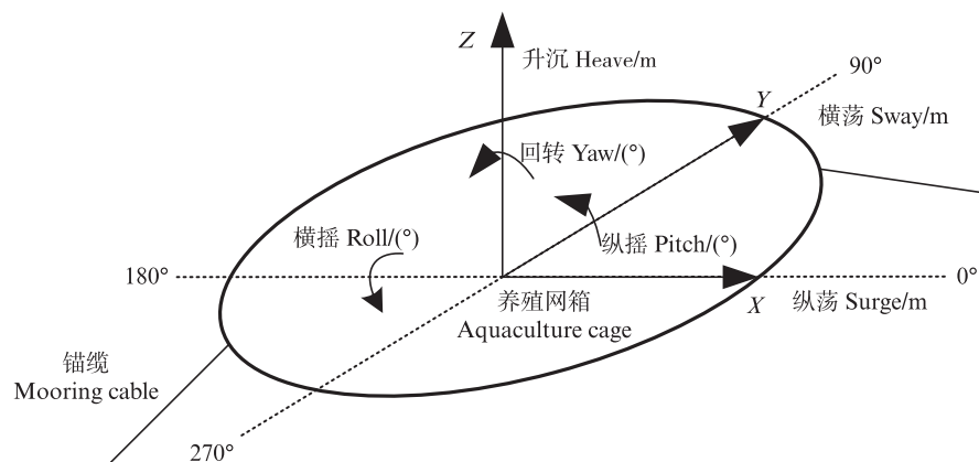
图5 养殖网箱6自由度
