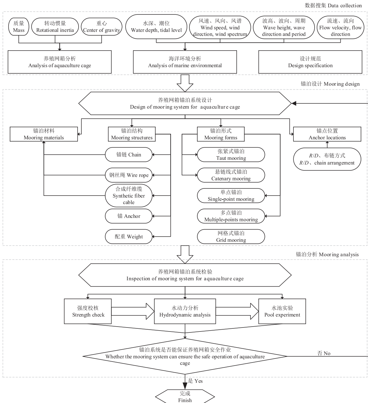
图 6 养殖网箱锚泊系统设计思路
